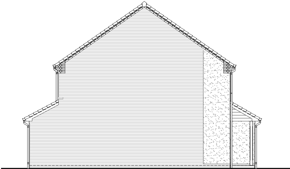
Right Elevation
